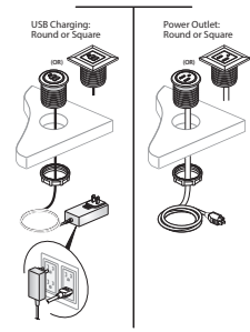
Bezel Utility Module
