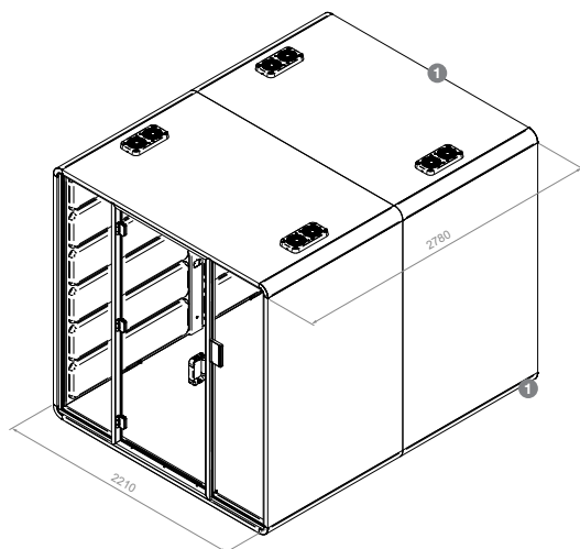
1 Accès au câble d'alimentation
