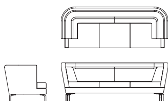
ENT/5/L Canapé trois places (dossier bas)
